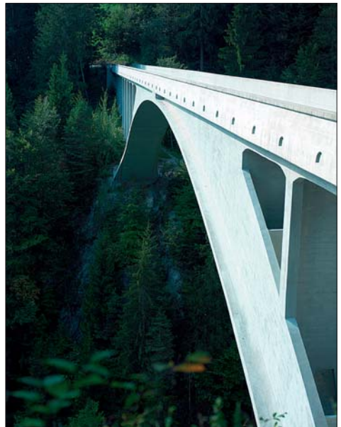
■ Salginatobelbrücke, Worldmonument, Schiers im Prättigau, Graubünden (Robert Maillart, Konstrukteur, 1929–1930)
